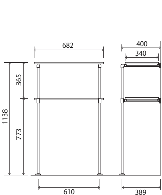
S-2 ¥14,000 2 段ラック
