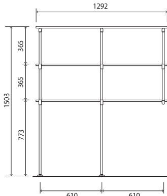
WLR-33 ¥38,000 3 段ラック+3 段カウンター脚なし
