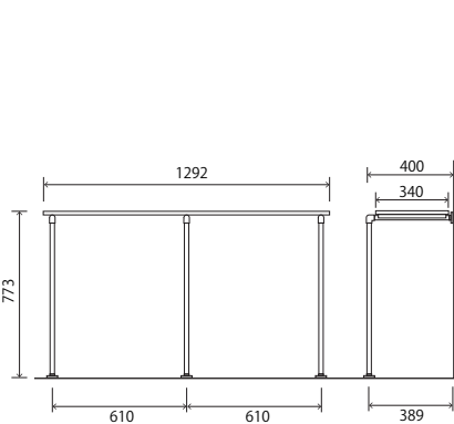
W-1 ¥14,000 1 段ラック W
