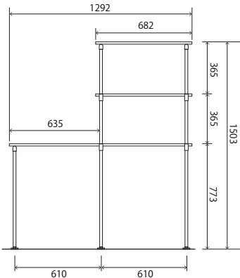
WL-31R ¥28,000 3 段ラック+カウンター R (反転タイプ)
