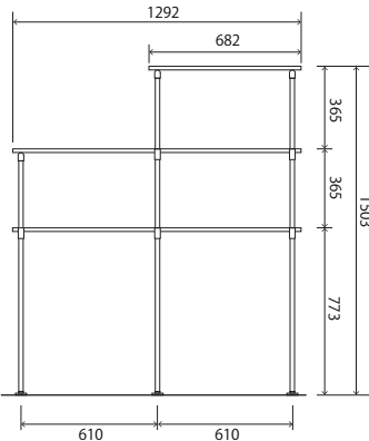
WL-32R ¥33,000 3 段ラック+2 段カウンター R (反転タイプ)
