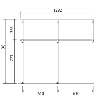
WLR-22 ¥28,000 2 段ラック+2 段カウンター脚なし
