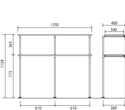
W-2 ¥28,000 2 段ラック W
