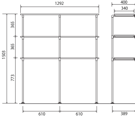
W-3 ¥38,000 3 段ラック W
