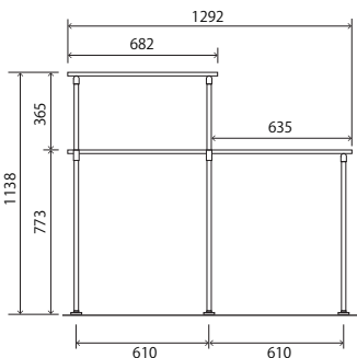
WL-21 ¥24,000 2 段ラック+カウンター
